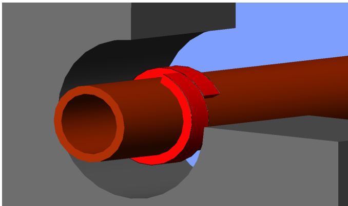
Rys. 3. Montaż taśmy Swell Sil w przepuszczeniu rury przez przegrodę.
